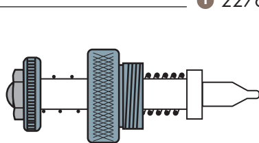
Percuteur complet
