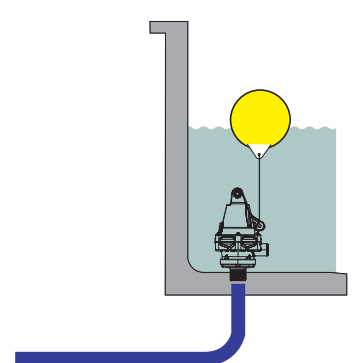
Montage hors gel par le dessous ficelle courte, pour un niveau plus bas
