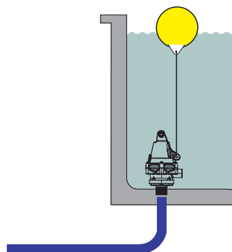
Montage hors gel par le dessous ficelle longue
