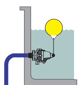
Montage sur le côté ficelle courte, pour un niveau plus bas
