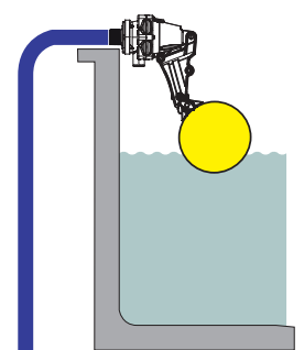
Entrée en haut avec extension
