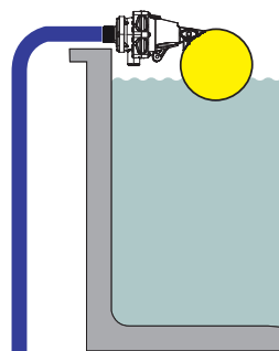
Entrée en haut sans extension
