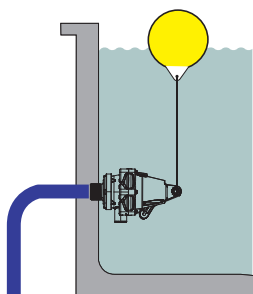
Montage sur le côté ficelle longue
